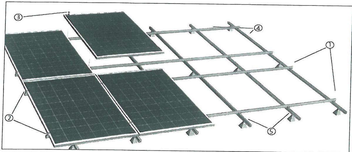
Budowa systemu
